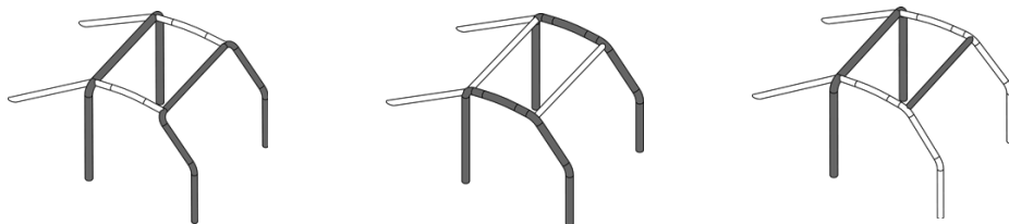
Pääkaarien taivutustavat kuvat 253-1, 253-2 ja 253-3.
